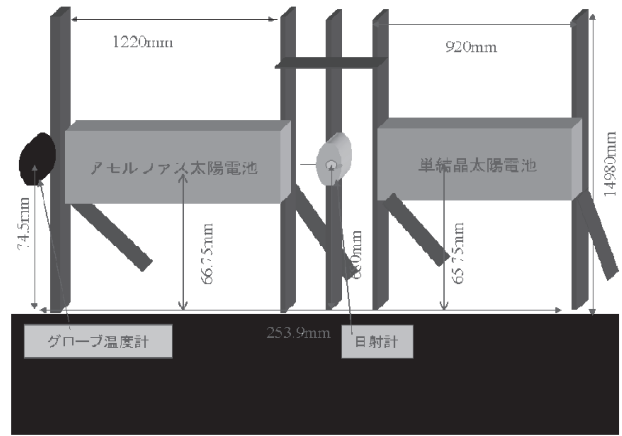
図3 実験装置図（雪面反射無し）
