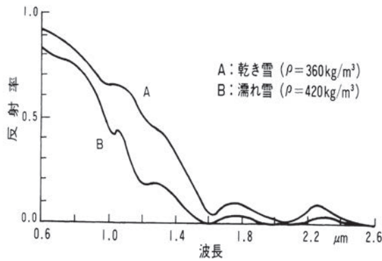
図10 積雪の波長別反射率 8)
