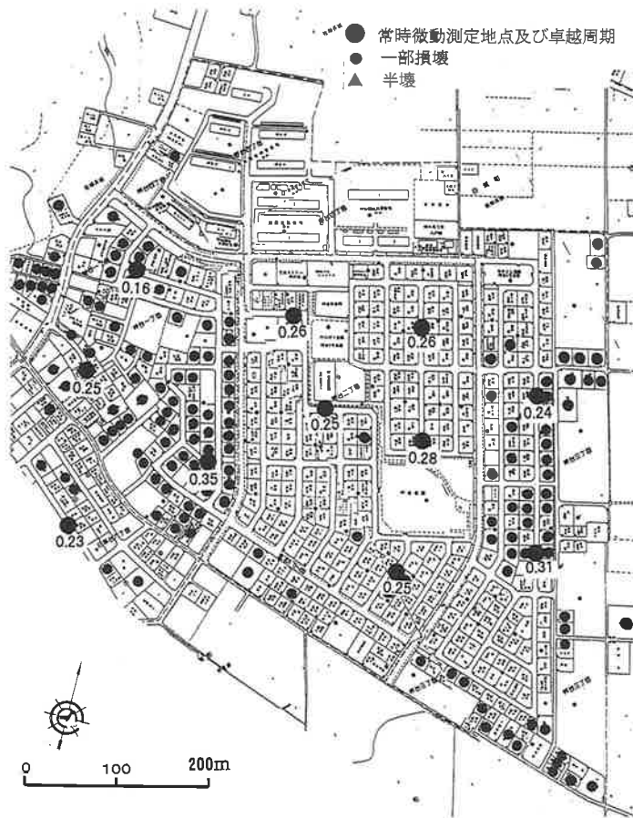
図2(3) 住宅被害分布と測定地点の卓越周期 岬台
