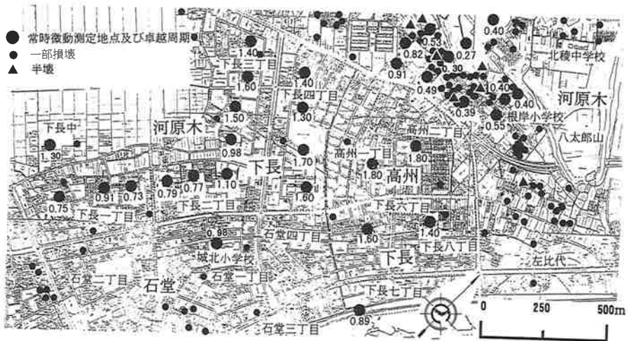
図2(4) 住宅被害分布と測定地点の卓越周期 下長
