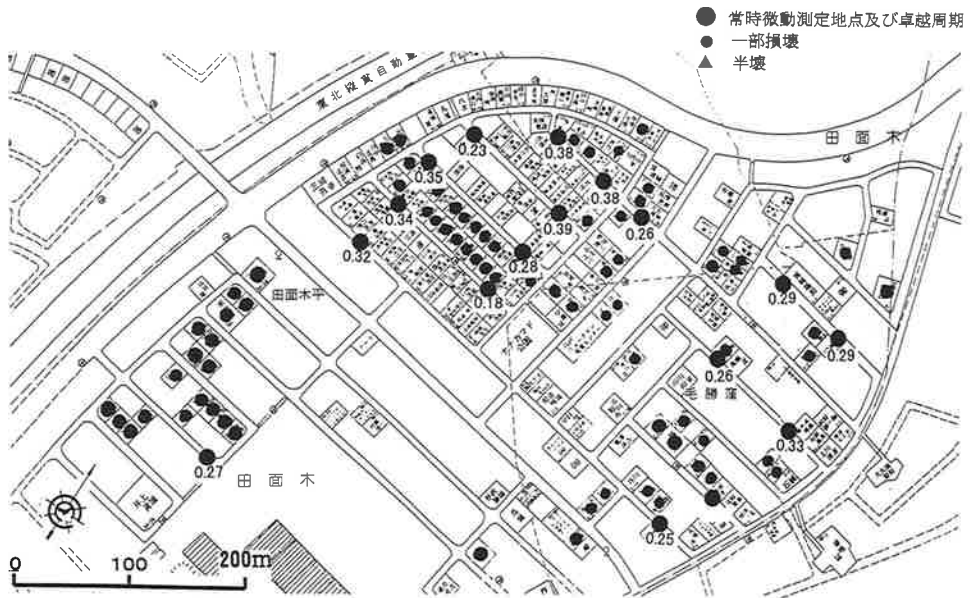
図 2(2) 住宅被害分布と測定地点の卓越周期 八戸ニュータウン
