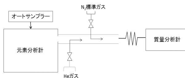
Fig.5 δ 15 N測定機器構成図
