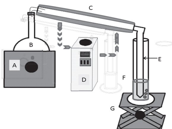
Fig.4 アンモニア蒸留装置
