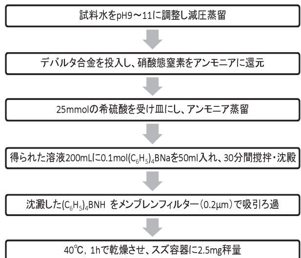
Fig.2 前処理工程
