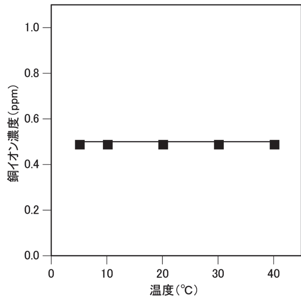
図7 EM 活性液を用いた銅イオン濃度に及ぼす溶液温度の影響
