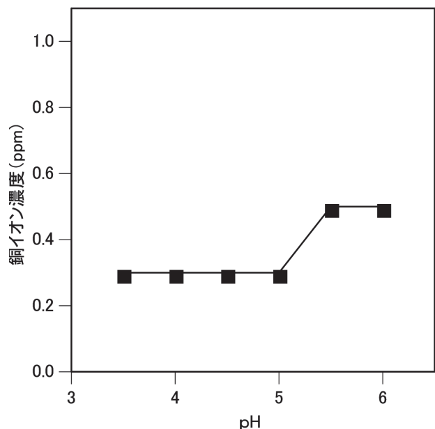
図 2 納豆懸濁液処理における銅イオン濃度に及ぼす pH の影響
