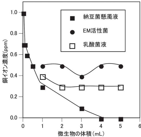
図 12 微生物処理における銅イオン濃度に及ぼす微生物液の体積の影響
