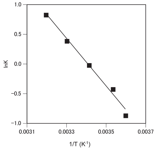
図11 乳酸菌液処理における銅イオン吸着平衡に及ぼす温度の影響に対するVan't Hoffプロット
