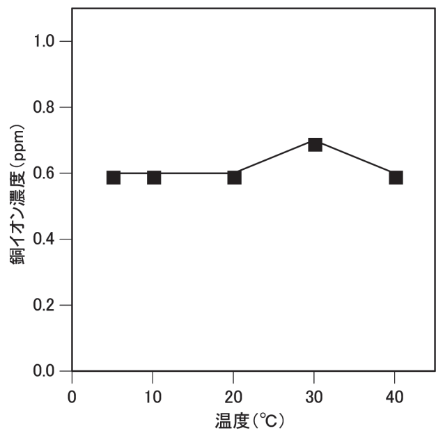
図4 納豆菌懸濁液処理における銅イオン濃度に及ぼす溶液温度の影響
