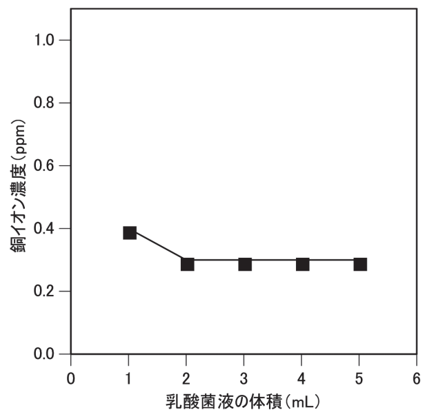
図8 乳酸菌液処理における銅イオン濃度に及ぼす乳酸菌液の体積の影響
