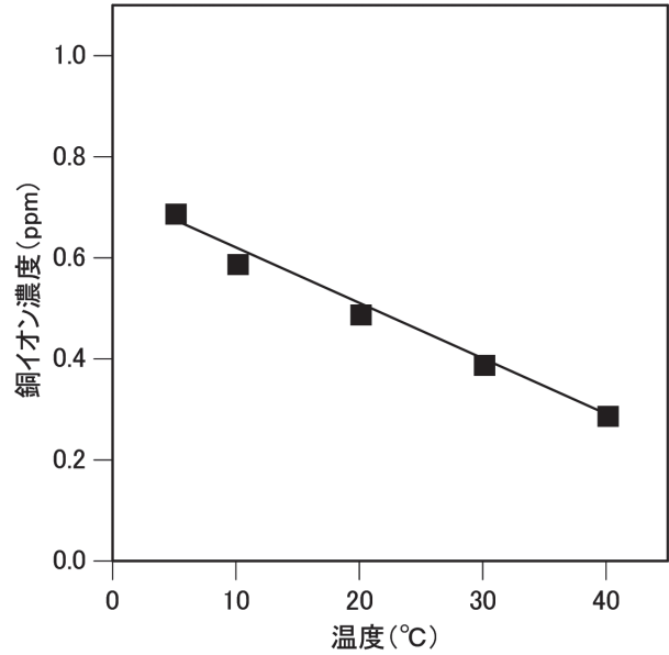
図10 乳酸菌液処理における銅イオン濃度に及ぼす溶液温度の影響
