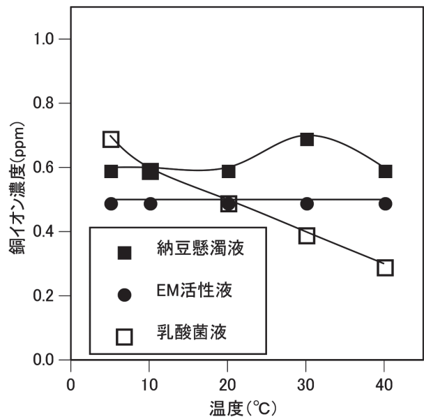
図 14 微生物処理における銅イオン濃度に及ぼす温度の影響
