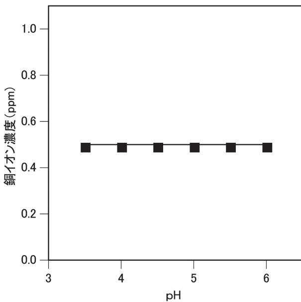
図6 EM 活性液処理における銅イオン濃度に及ぼす pH の影響
