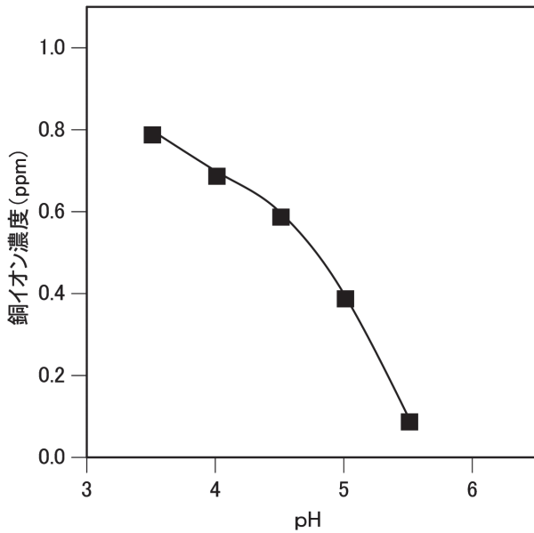
図9 乳酸菌液処理における銅イオン濃度に及ぼすpHの影響
