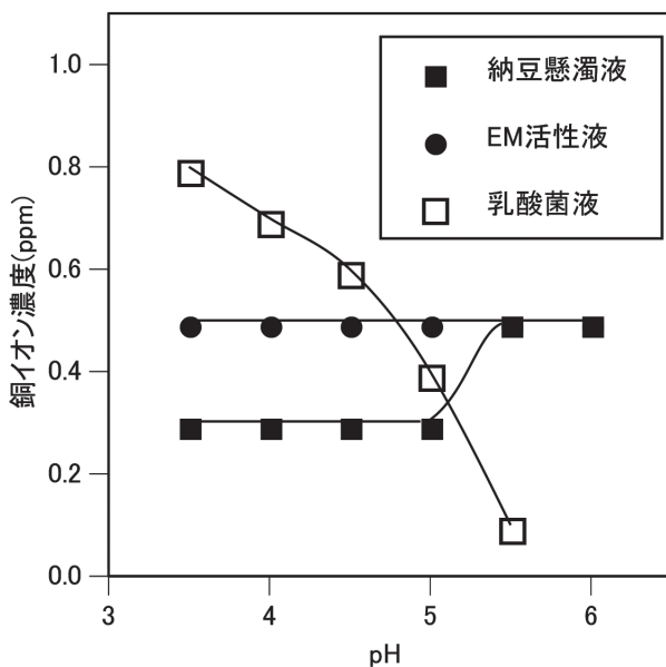
図 13 微生物処理における銅イオン濃度に及ぼす pH の影響
